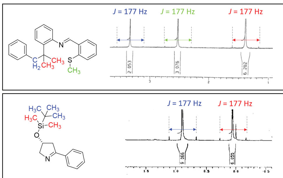
Слика 4. Репродукција делова ^1\text{H} НМР-спектара датих за једињења 2 и 4 . Означене су константе спрезања ^1\text{H} - ^{13}\text{C} кроз једну везу, а различите боје дате су у сврху асигнације
