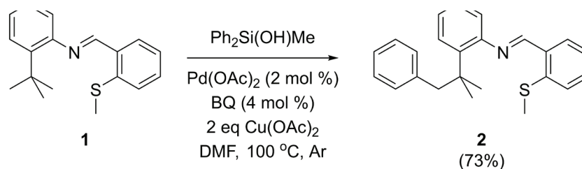
Схема 1. Каталитичко ариловање Шифове базе 1 дифенилметилсиланолом (Sezen et al., 2002); Ph = фенил, Ac = ацетил, BQ = бензохинон, DMF = N,N -диметилформамид
