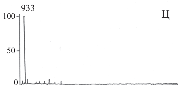
Слика 5. МАЛДИ-ТОФ МС анализа укупног серумског Н-гликома (десијалинизованог) здраве особе након дигестије егзогликозидазама (преузето из [5]). А) серум третиран \beta -галактозидазом, Б) серум третиран комбинацијом \beta -галактозидазе и \beta -Н-ацетилхексозаминидазе и Ц) серум третиран комбинацијом \beta -галактозидазе, \beta -Н-ацетилхексозаминидазе и \alpha -фукозидазе.
