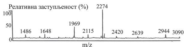
Слика 4. МАЛДИ-ТОФ МС анализа укупног серумског Н-гликома здраве особе (гликани су метиловани, Me). Главни пик на m/z 2274 одговара гликану састава \text{SiaMe}_2\text{Hex}_5\text{HexNAc}_4 , док веома сличан гликан, само са једним остатком Sia даје пик на m/z 1969 ( \text{SiaMeHex}_5\text{HexNAc}_4 ). Одговарајући гликани са остатком L-Fuc у језгру гликана примећени су на m/z 2420 ( \text{SiaMe}_2\text{Hex}_5\text{HexNAc}_4\text{DeoxyHex} ) и 2115 ( \text{SiaMeHex}_5\text{HexNAc}_4\text{DeoxyHex} ). Преузето из [5].
