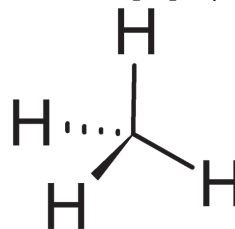
Слика 2. Структурна формула метана.
